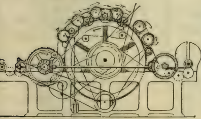
( پاموق ماکنه سی )
